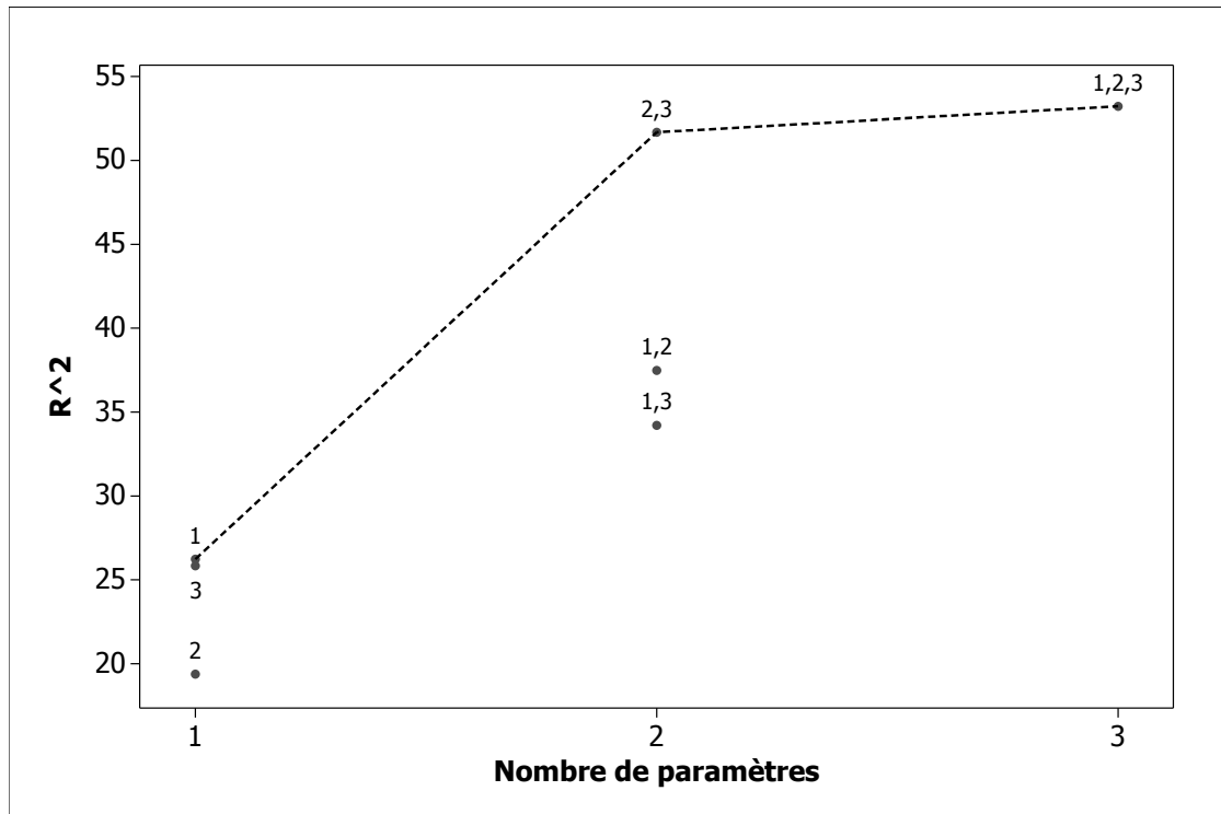
FIG. 1. Graphique des R^2
