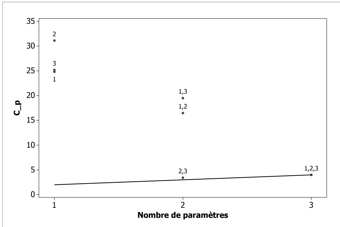
FIG. 3. Graphique des C_p
