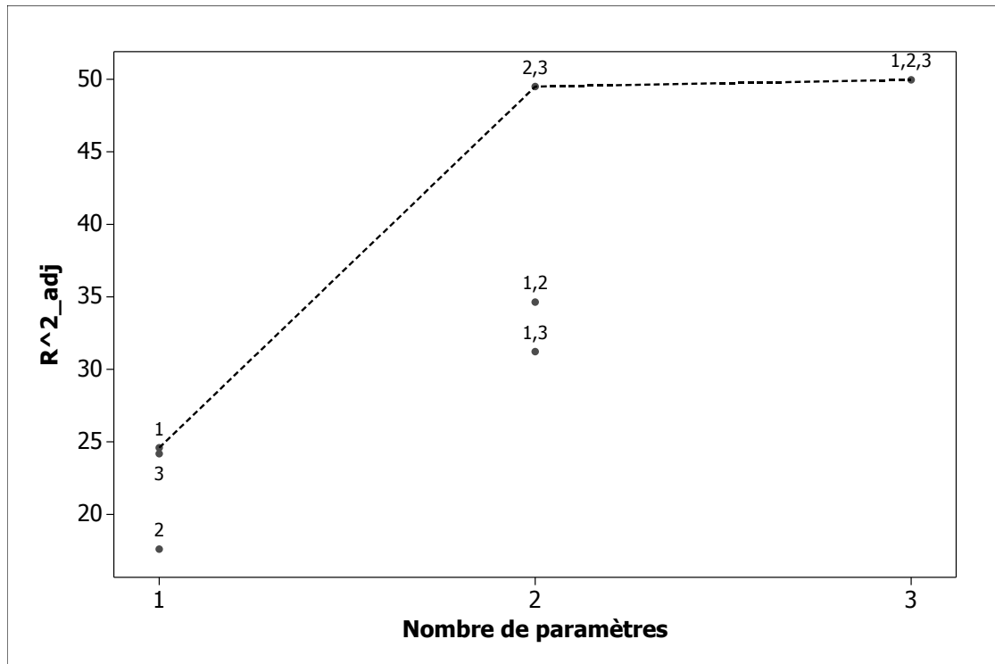
FIG. 2. Graphique des R^2 ajustés
